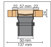
Querschnitt Miteleinbau
