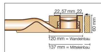
Querschnitt
