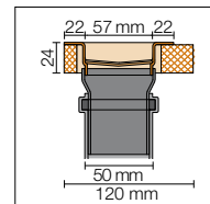
Querschnitt Wandeinbau
