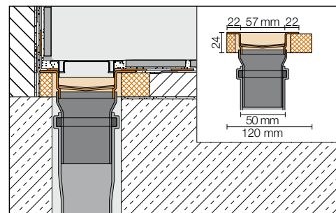
Schlüter®-KERDI-LINE-V
