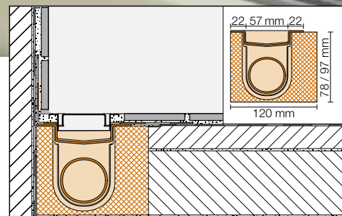
Schlüter®-KERDI-LINE-H
