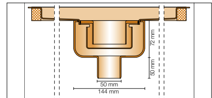
Längsschnitt Wand- /Miteleinbau
