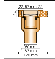
Querschnitt Wandeinbau
