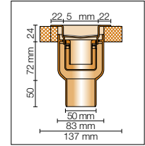
Querschnitt Miteleinbau
