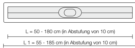
Längsschnitt Wand- /Miteleinbau
