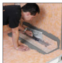
zu 4. KERDI-Manschette mit KERDI-COLL aufkleben
