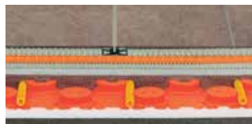
Aufbau mit Schlüter®-BEKOTEC-EN/P bzw. -EN/PF
